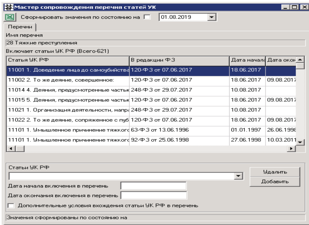
Рис. 4. Экранная форма ввода (вывода) статей УК РФ в перечень
